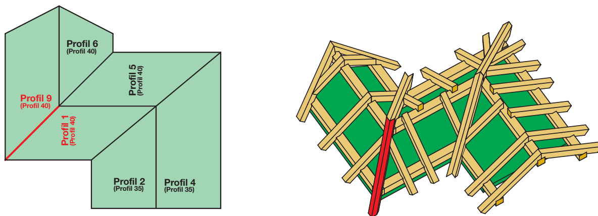
Bild 33: Die Dachausmittlung. Der Gratsparren Pos. 14 liegt zwischen Profil 9 und Profil 1.
