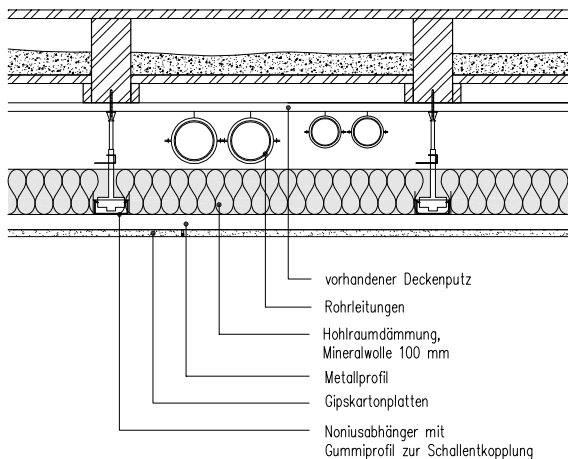
Abb. 5.10: Zusätzliche Unterdecke mit Hohlraum für Installationen (Noniusabhängiger)
